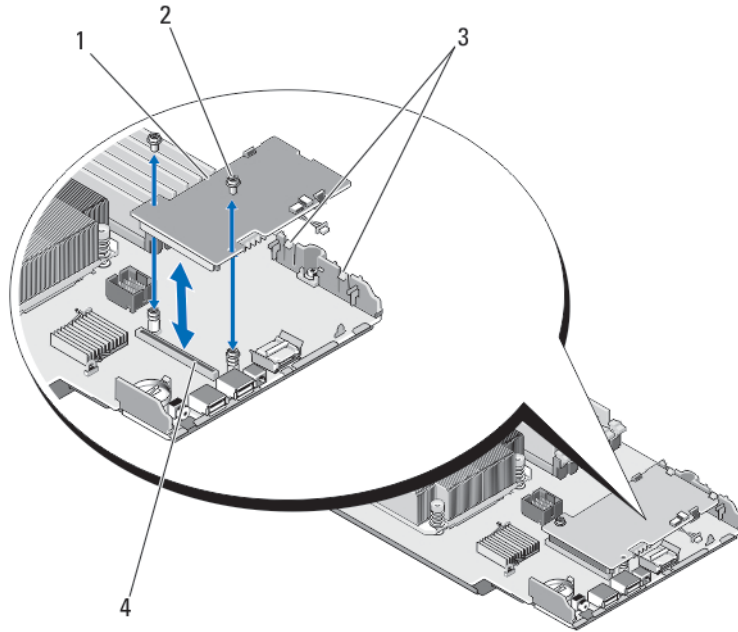
그림 22. 저장소 컨트롤러 카드 분리 및 설치
