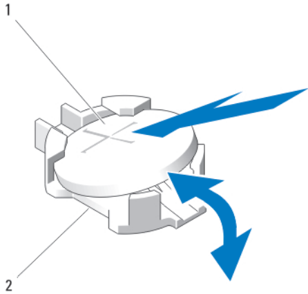
그림 21. NVRAM 백업 전지 장착
