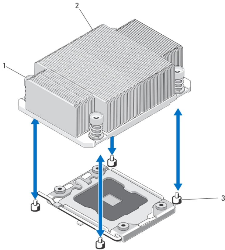
그림 15. 방열판 분리 및 설치
