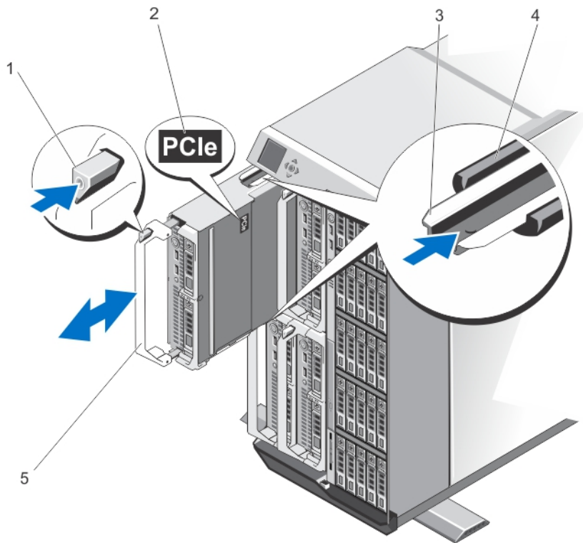
그림 5. 서버 모듈 분리 및 설치
