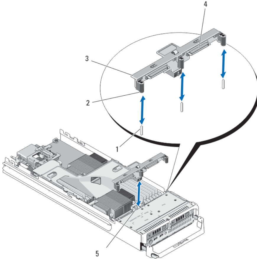
그림 19. 하드 드라이브/SSD 후면판 분리 및 설치
