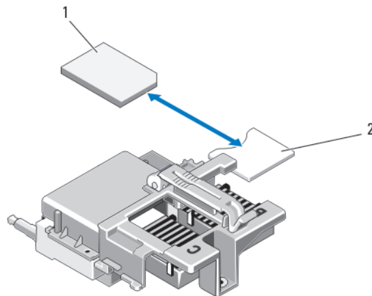
그림 14. SD vFlash 카드 장착
