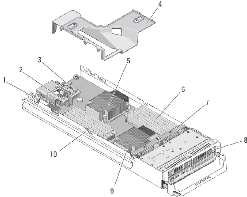
그림 7. 서버 모듈 내부
