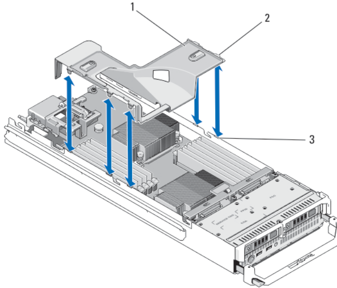
그림 8. 냉각 덮개 분리 및 설치
