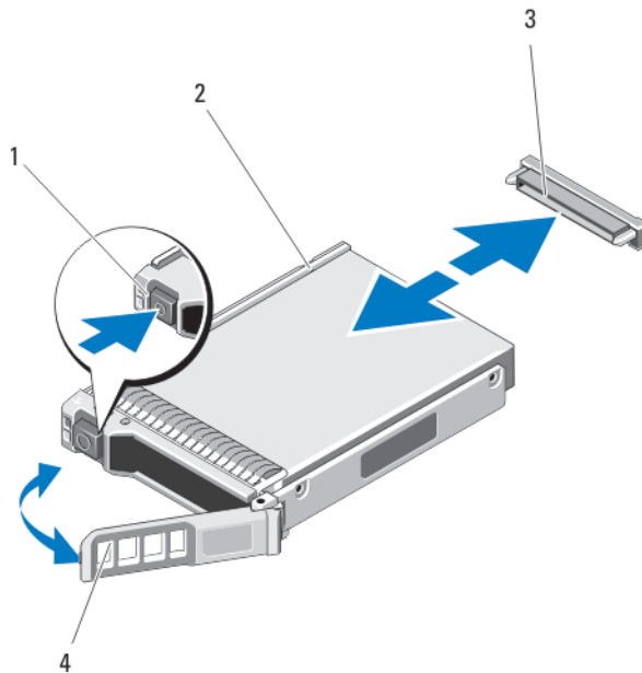
그림 17. 하드 드라이브/SSD 분리 및 설치
