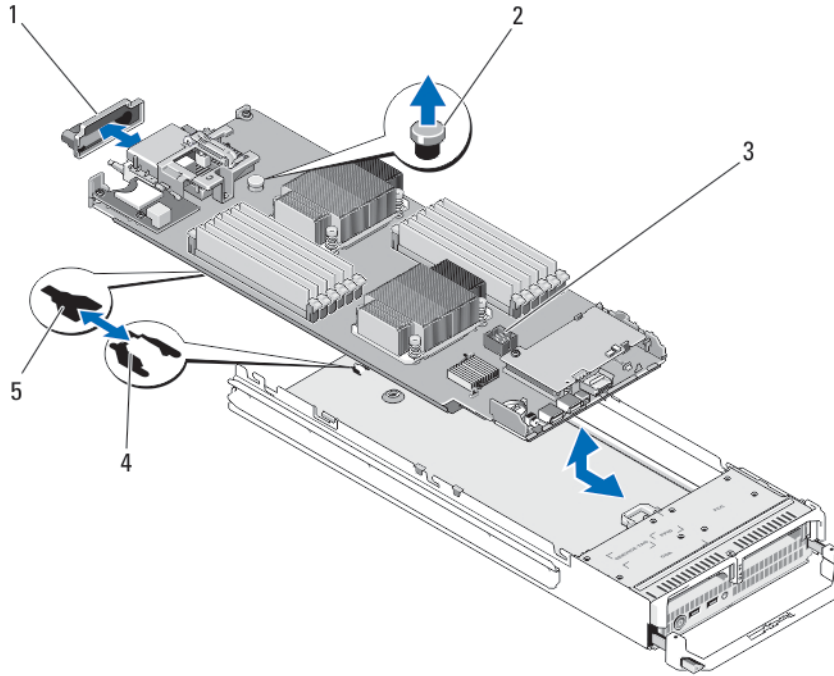
그림 20. 시스템 보드 분리 및 설치
