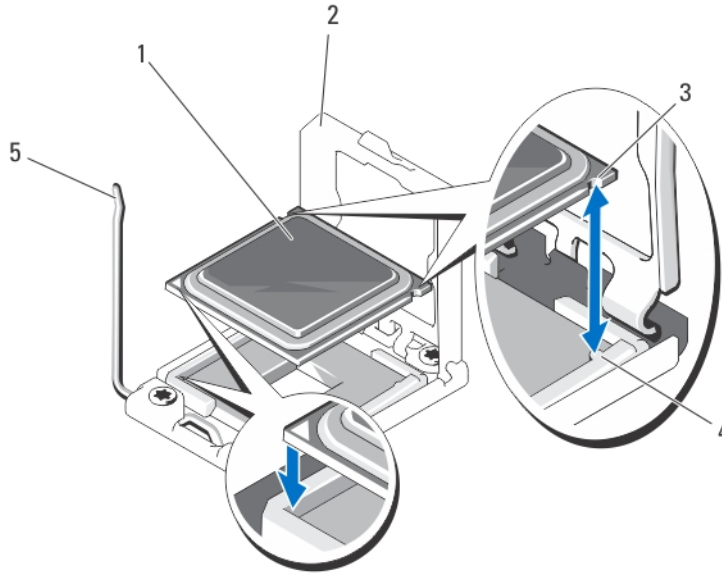
그림 16. 프로세서 분리 및 설치
