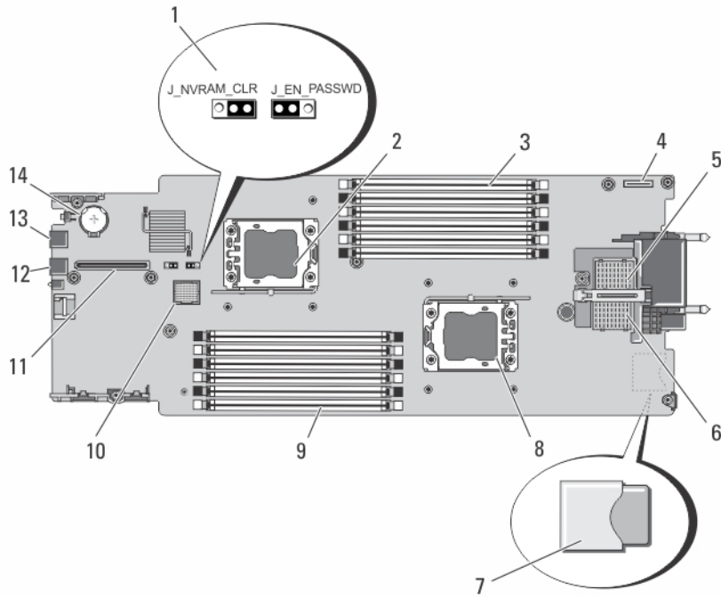
그림 23. 시스템 보드 커넥터
